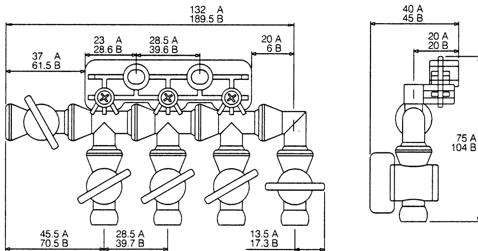
Mehrfachverteiler 21198 & 32098
