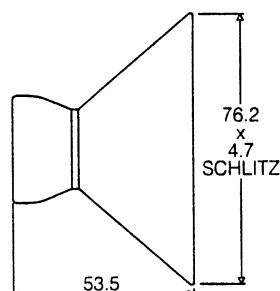
Flachdüse 61507
