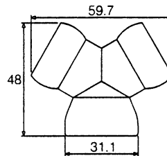
3/4" Gelenkstücke 61501
