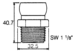
Gewindenippel 3/4" 61505
