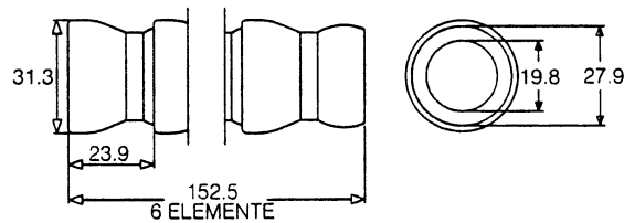
3/4" Gelenkstücke 61501
