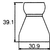
Reduktion 19/12mm 61508
