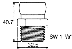
Gewindenippel 3/4" 61509
