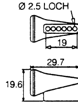
Mehrlochwinkeldüse 41473
