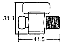
Kugelhahn 1/4" Aussengewinde 21192
