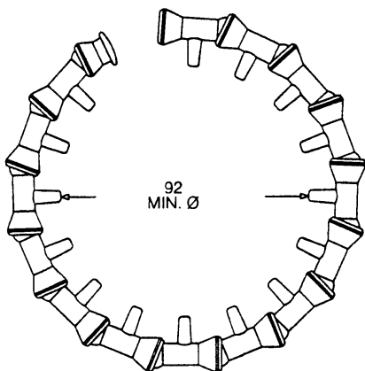
Ringdüsensatz 41479
