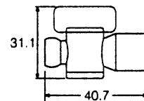
Kugelhahn 1/4" Innengewinde 21193
