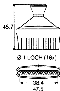
Mehrloch-Schwenkdüse 41481
