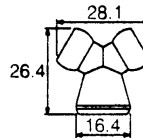
Y-Abzweigstück 41408
