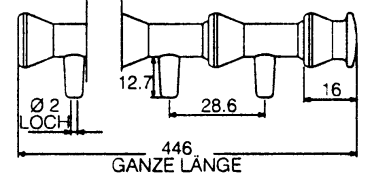
T-Düsen 41479
